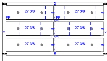
VLT-1021D-60 60"W x 35"H x 21½"D
