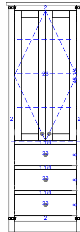
LLT-1023-27 27"W x 84"H x 24"D
