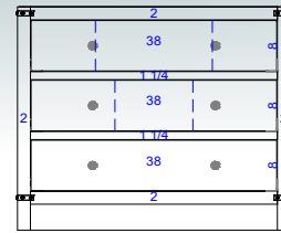
VLT-1021-42 42"W x 35"H x 21½"D
