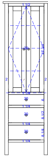
LCA-323-24 24"W x 84"H x 24"D
