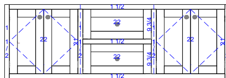
VFI-1241D-72 72"W x 24"H x 21"D
