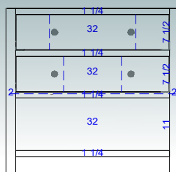
VOS-141-36 36"W x 35"H x 21 1/2"D
